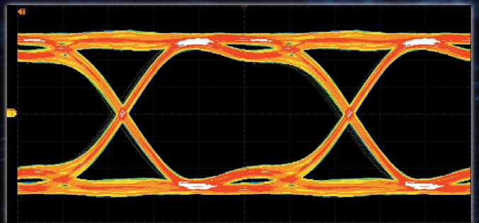
使用600 MHz带宽和2 GHz带宽分别对1 Gb/s信号进行眼图观测
