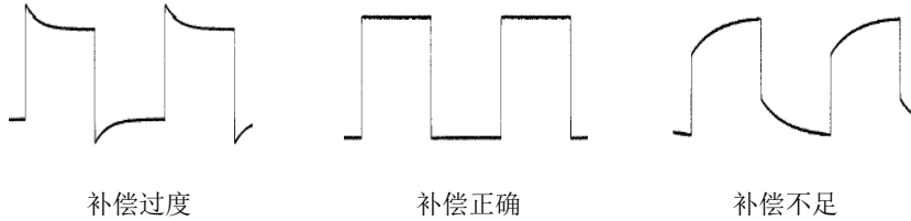
图 8 探头补偿
